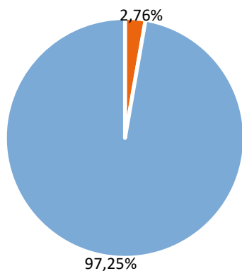
Triedy aktív
